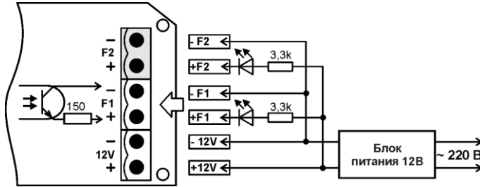
Рисунок 23 – Контроль выходных сигналов P542_1352
