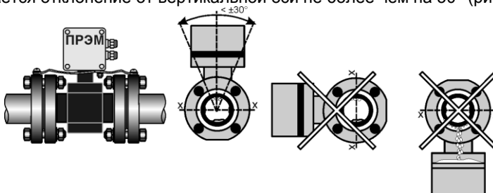
Рисунок 12 – Установка на горизонтальных каналах
